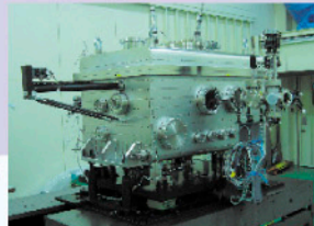
Monochromator (DEIMOS)
